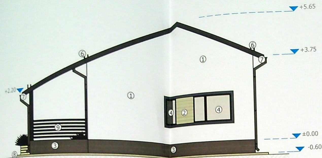
FATADA EST scara 1:100
