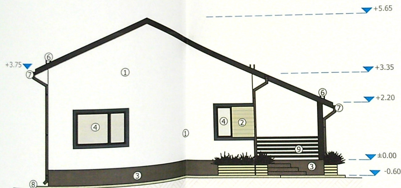
FATADA VEST scara 1:100
